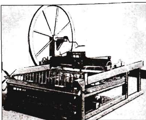
Hình 61 – Máy Gien-ni
